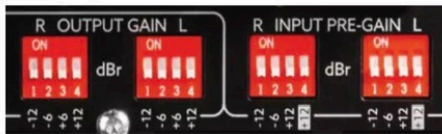
MÄUSE-KLAVIER: Die Pre-Gain der Eingänge und die Ausgangsverstärkung lassen sich auf der Rückseite anpassen.
